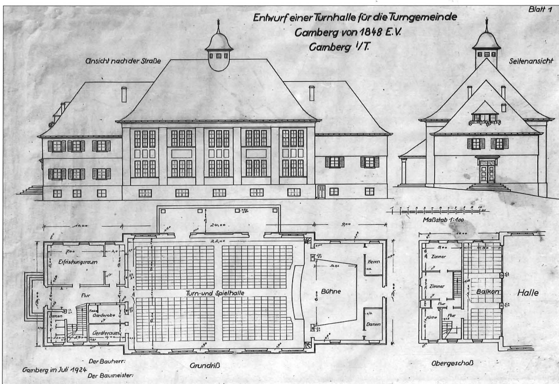
Entwurf der geplanten Turnhalle, 1925
